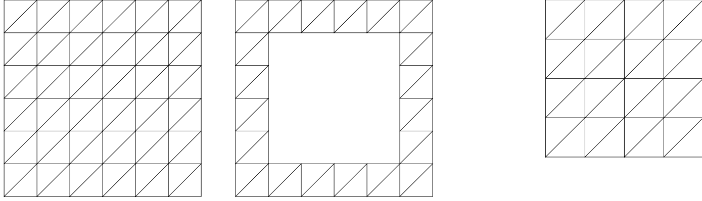
Maillage T du domaine \Omega Mailles fictives Maillage total
